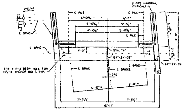
PLAN SCALE: 1/4" = 1'-0"
