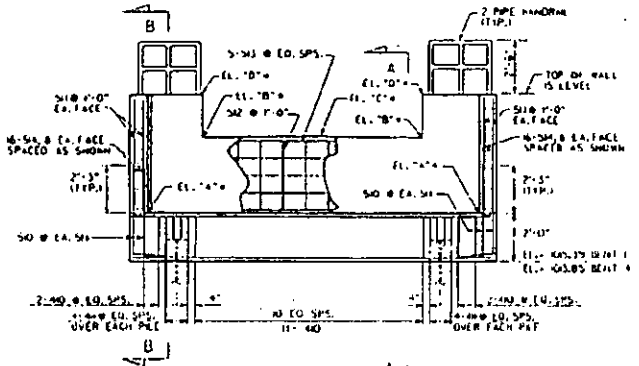
ELEVATION SCALE: 1/4" = 1'-0"
